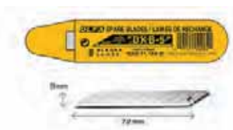
Rezervni nož. DKB-5
